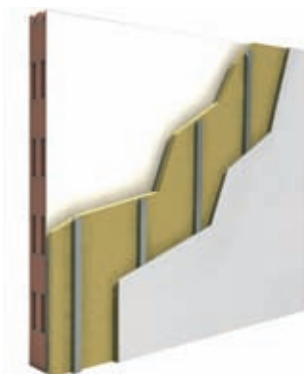
Controparete ad orditura metallica vincolata alla muratura esistente
